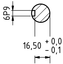
B-B ( 1 : 2 )
