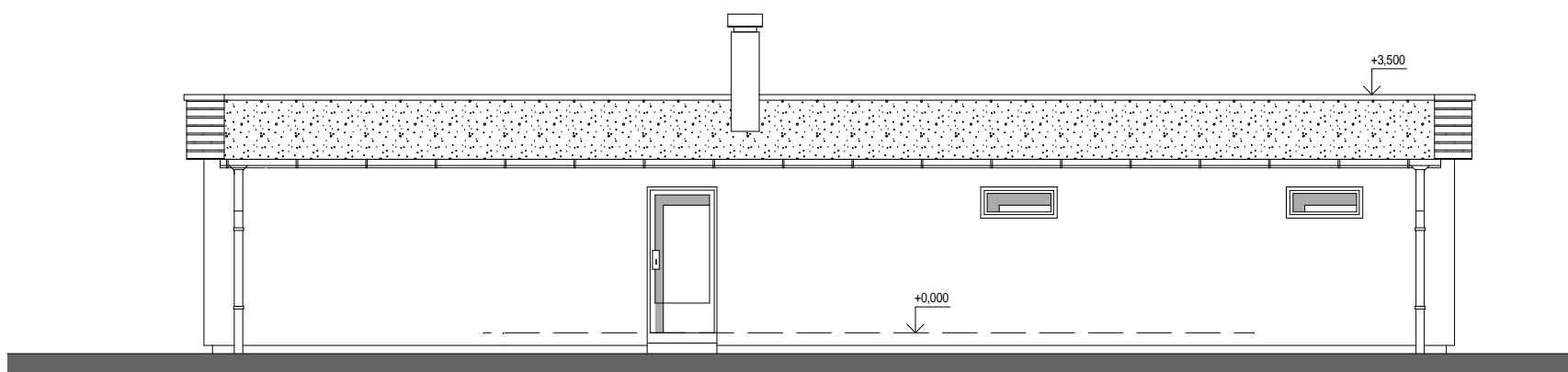
POHLED ČELNÍ se VSTUPEM
