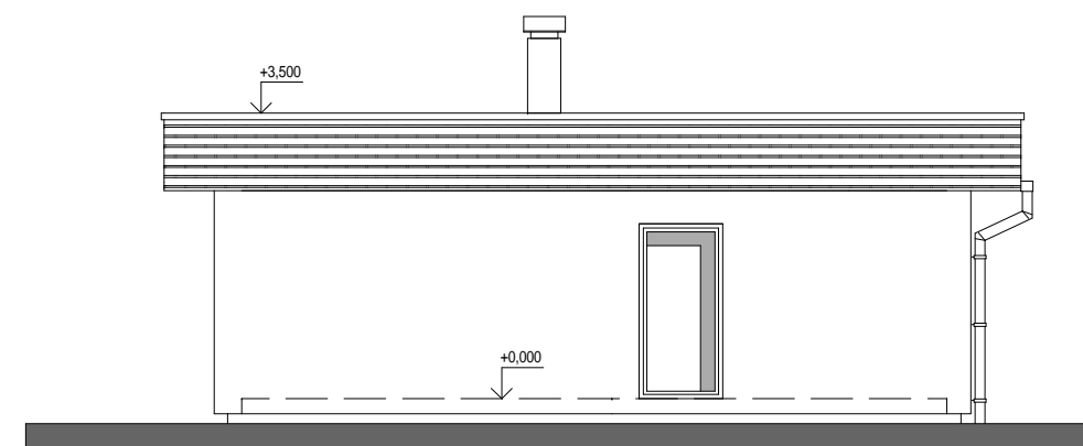
POHLED BOČNÍ 1
