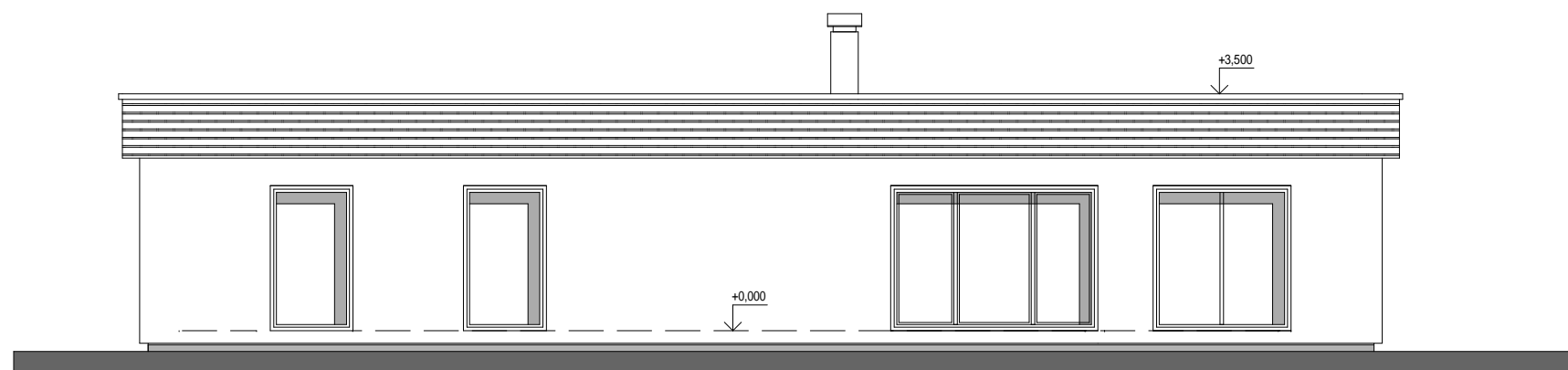
POHLED ZADNÍ s TERASOU
