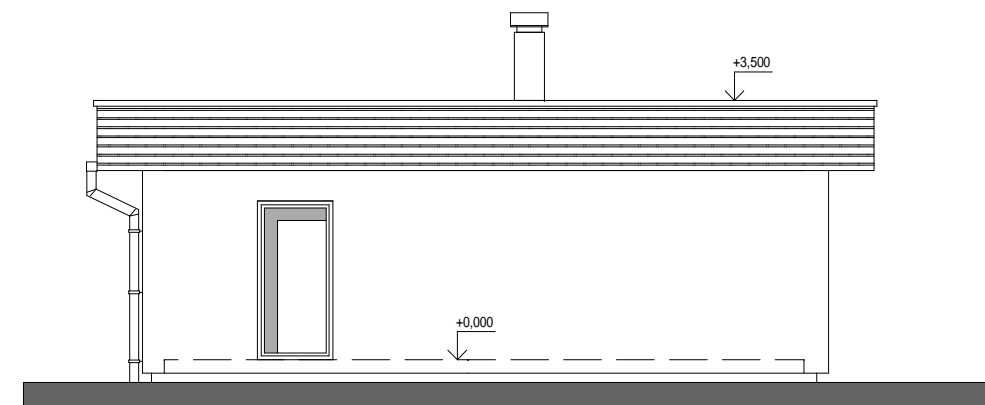
POHLED BOČNÍ 2
