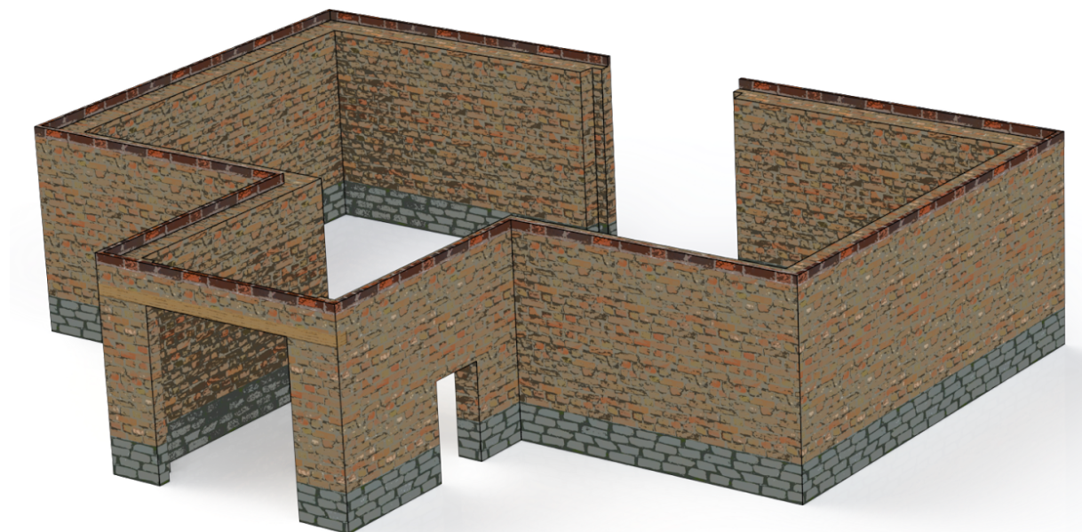
Obrázok č.1: CAD model obvodových múrov stodoly (ilustračný účel)
