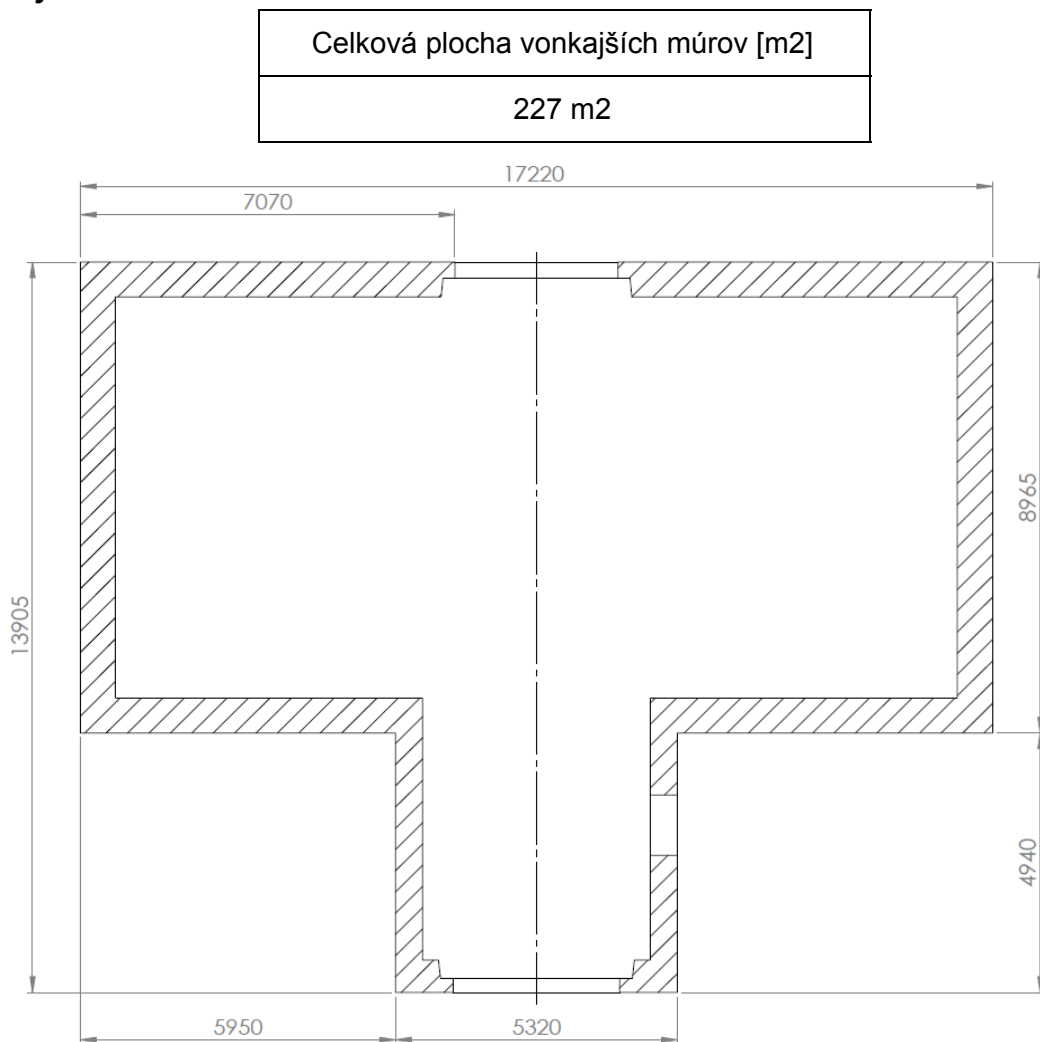
Obrázok č.2: Rozmery obvodových múrov stodoly (v milimetroch)
