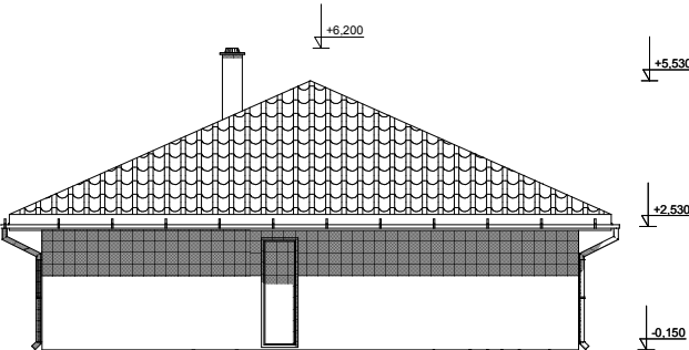
Pohled severovýchodní a jihovýchodní, M 1:100
