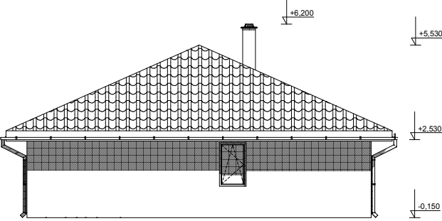
Pohled jihozápadní a severozápadní, M 1:100
