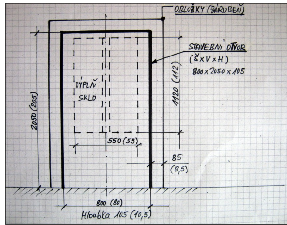
Zaměření (stavební otvor 800x2050x105)
