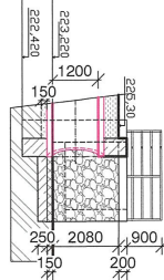
Řez osou potrubí - levý břeh
