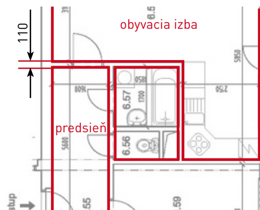
pôdorys
