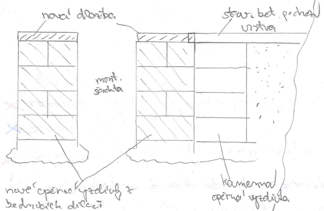
B-B ŘEZ
